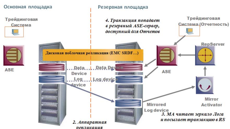
Рис. 2. Схема работы Mirror Activator в составе Sybase ASE.
